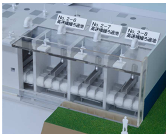
高速繊維ろ過装置 FIBAX（ジオラマ）
